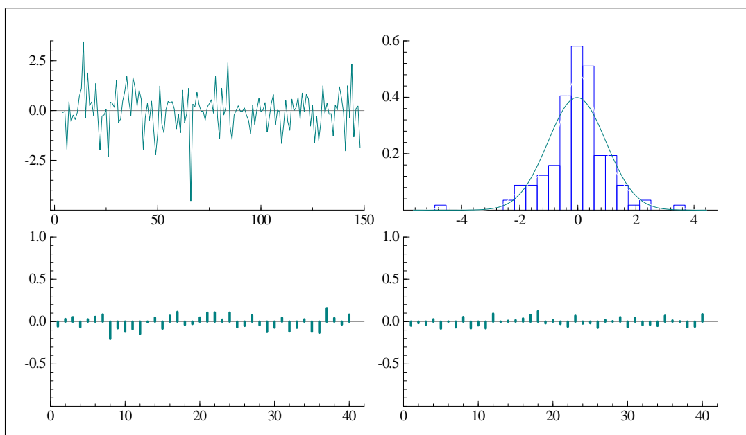
Kuvio 6.1. Kuvion 4.1 inflaatioasarjaan sovitetusta AR-GARCH-mallista (5.13) laskettu residuaalisarja (ylh. vas.), sen histogrammi ja N(0, 1) -jakauman tiheysfunktio (ylh. oik.) sekä residuaalien ja neliöityjen residuaalien otosautokorrelaatiofunktiot viipymillä h = 1, \dots, 40 (alh. vas. ja oik.).
