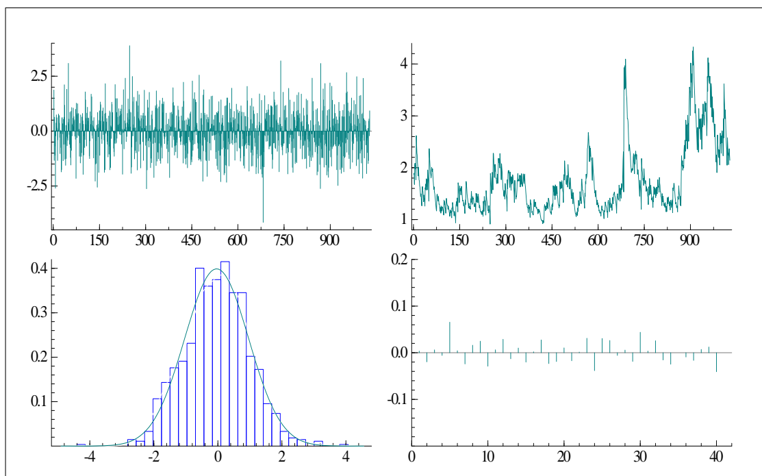
Kuvio 5.3. Kuvion 5.1 DAX-sarjaan sovitetusta GARCH(1,2)-mallista (5.14) laskettu residuaalisarja (ylh. vas.), sen histogrammi ja N(0, 1) -jakuman tiheysfunktio (alh. vas.), neliöityjen residuaalien otosautokorrelaatiofunktio viipymillä h = 1, \dots, 40 (alh. oik.) ja estimoitu ehdollinen hajonta \hat{h}_t^{1/2} (ylh. oik.).
