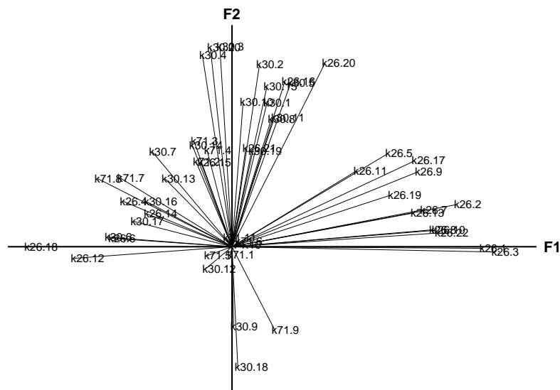
Kuva 4.2. Muuttujat faktoriavaruudessa.
